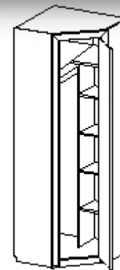
Шкаф угл.с пол. 77x77 шир./выс./глуб. 780x2170x780
