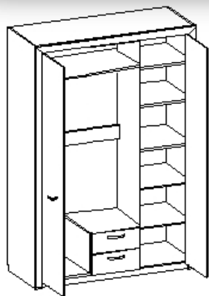
Корпус шкафа 3D2S шир./выс./глуб. 1360x2170x600
