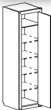
Шкаф 1DG шир./выс./глуб. 600x2170x600
