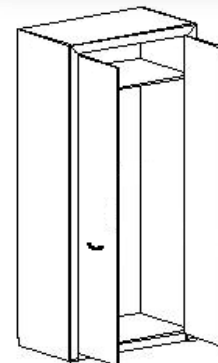
Шкаф 2DG шир./выс./глуб. 960x2170x600
